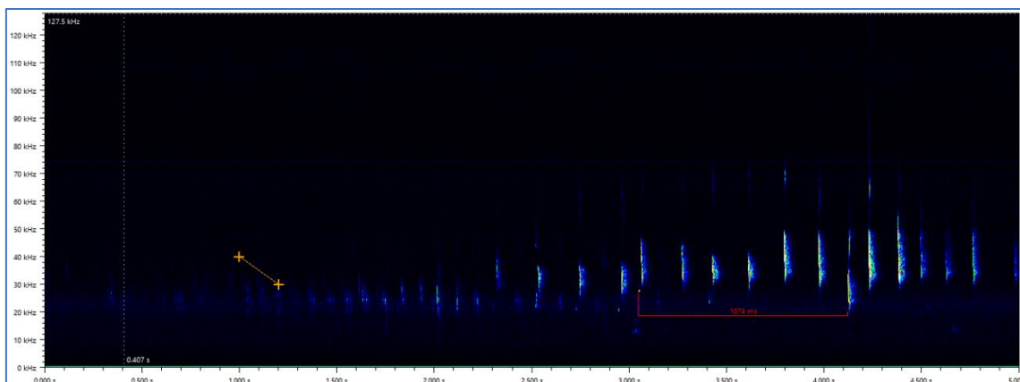
Figura 34. Sonograma de murciélago orejado gris ( Plecotus austriacus ) Fuente propia
