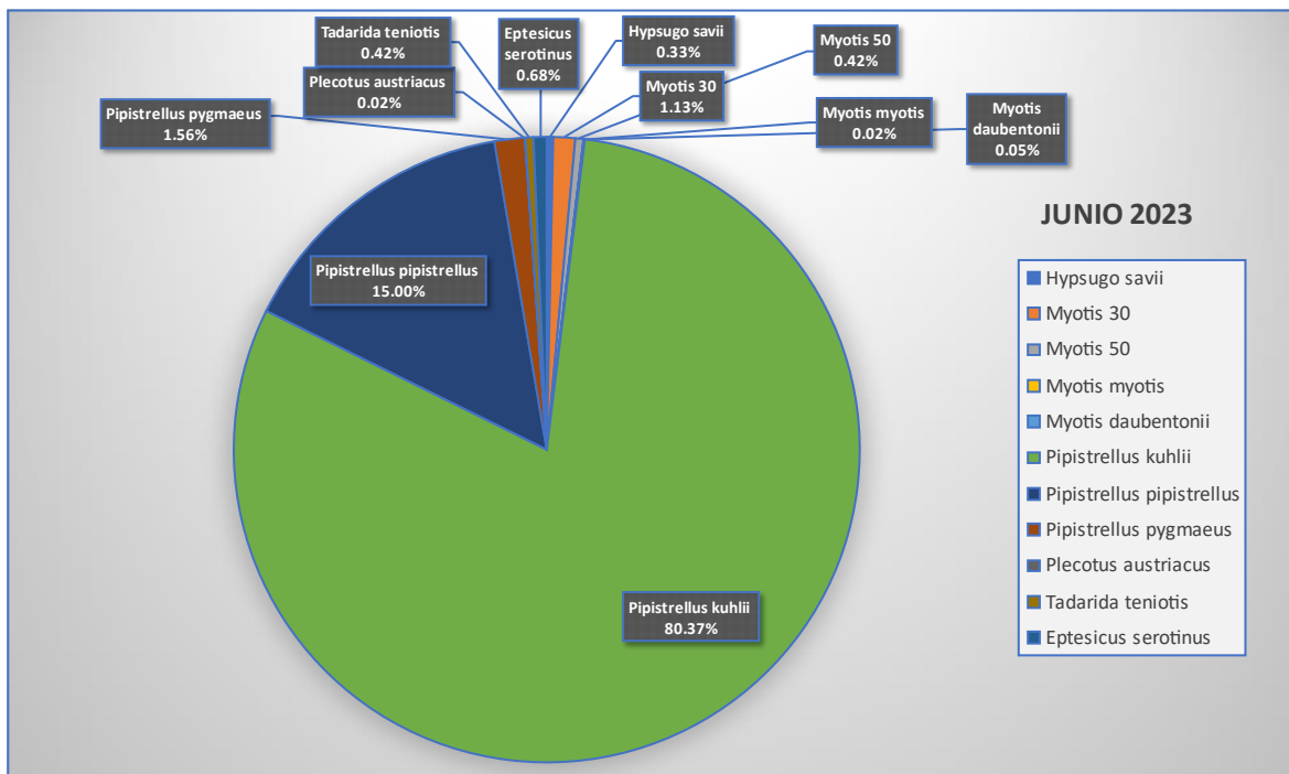
Figura 43. Distribución de todos registros obtenidos en la sesión del mes de junio de 2023 en la estación de ultrasonidos. Fuente propia
