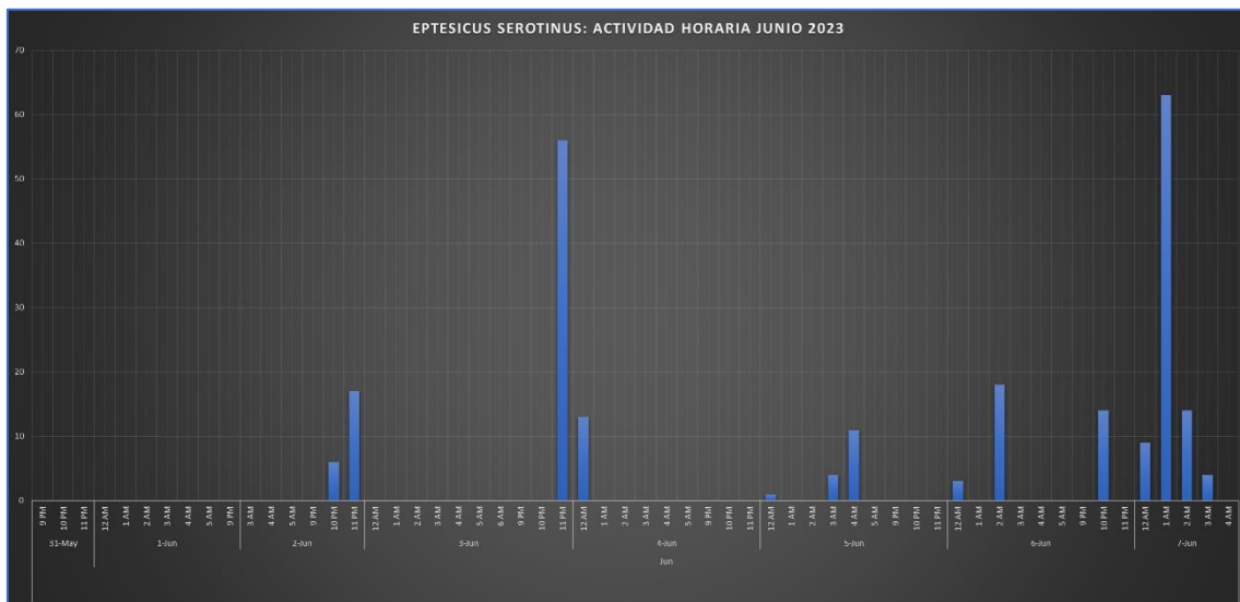
Figura 41. Actividad horaria de junio de Eptesicus serotinus . Fuente propia
