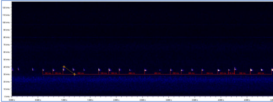
Figura 22. Sonograma de murciélago montañero ( Hypsugo savii ) Fuente propia
