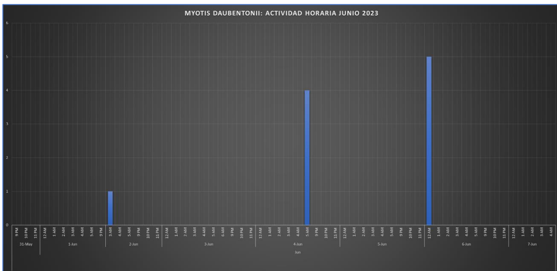
Figura 21. Actividad horaria junio del grupo fónico Myotis daubentonii . Fuente propia
