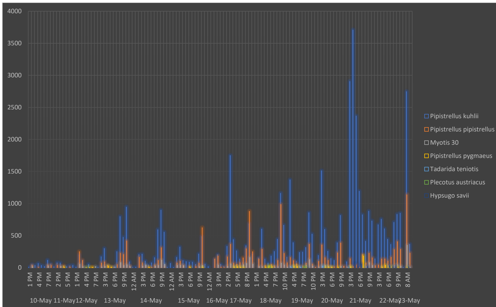
Figura 44. Distribución horaria de los registros obtenidos en la sesión del mes de mayo de 2023 en la estación de ultrasonidos. Fuente propia
