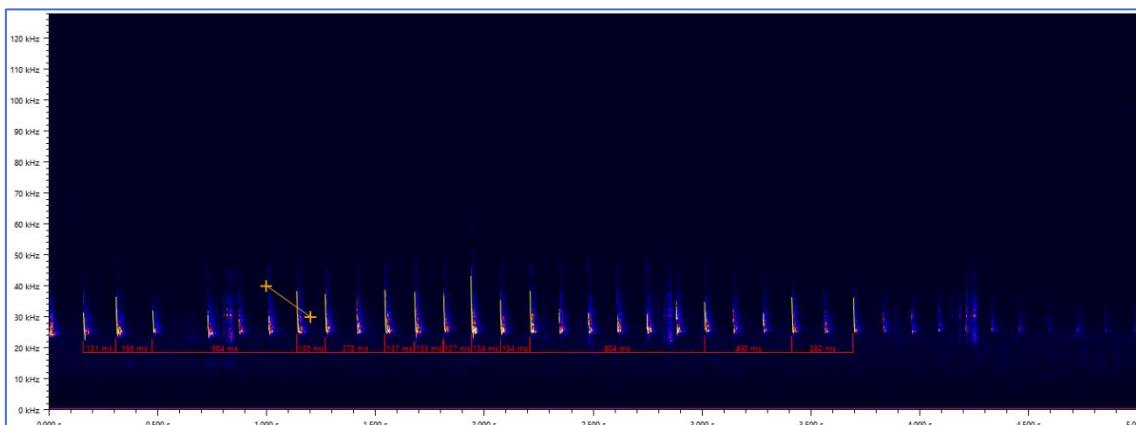
Figura 40. Sonograma de murciélagó hortelano ( Eptesicus serotinus ) Fuente propia
