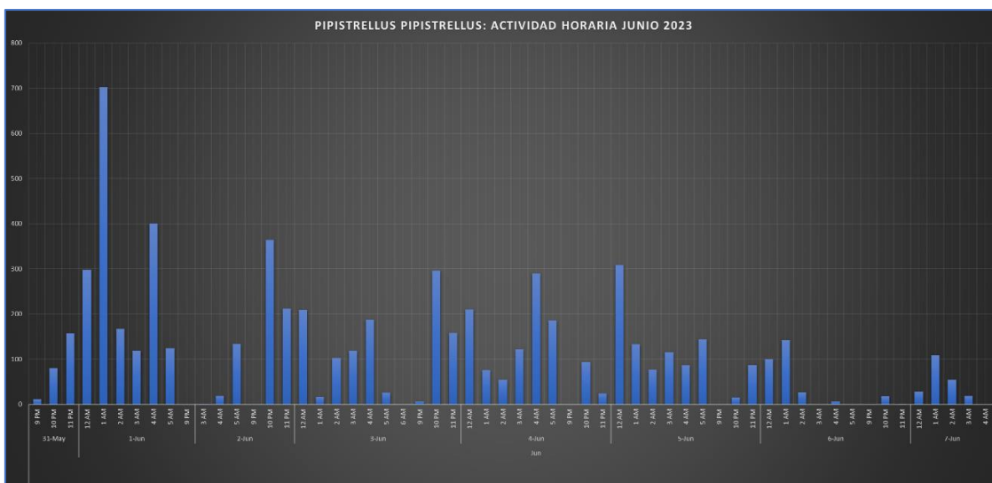
Figura 30. Actividad horaria de junio de Pipistrellus pipistrellus . Fuente propia
