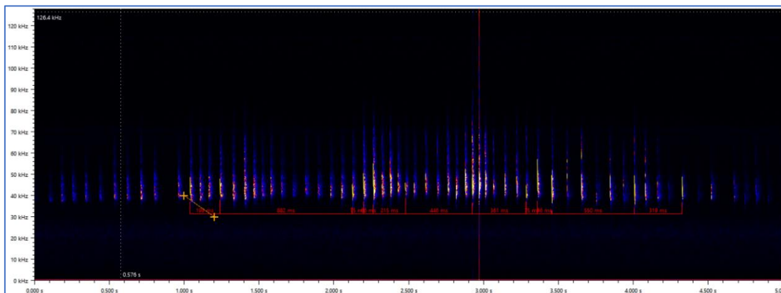
Figura 25. Sonograma de murciélagó de borde claro ( Pipistrellus kuhlii ) Fuente propia
