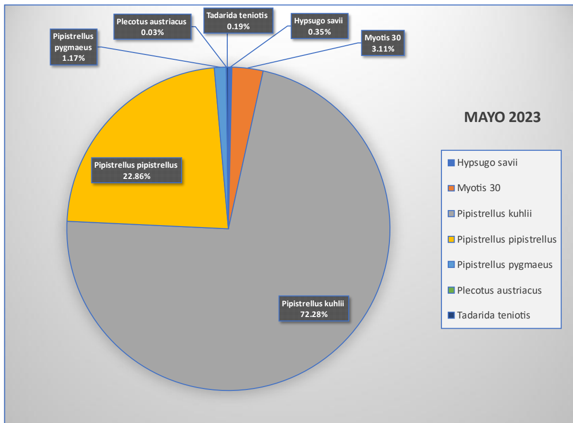
Figura 42. Distribución de todos registros obtenidos en la sesión del mes de mayo de 2023 en la estación de ultrasonidos. Fuente propia
