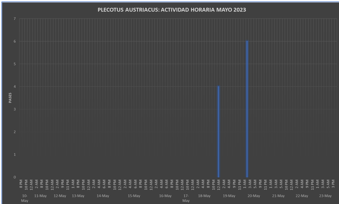
Figura 35. Actividad horaria de mayo de Plecotus austriacus . Fuente propia
