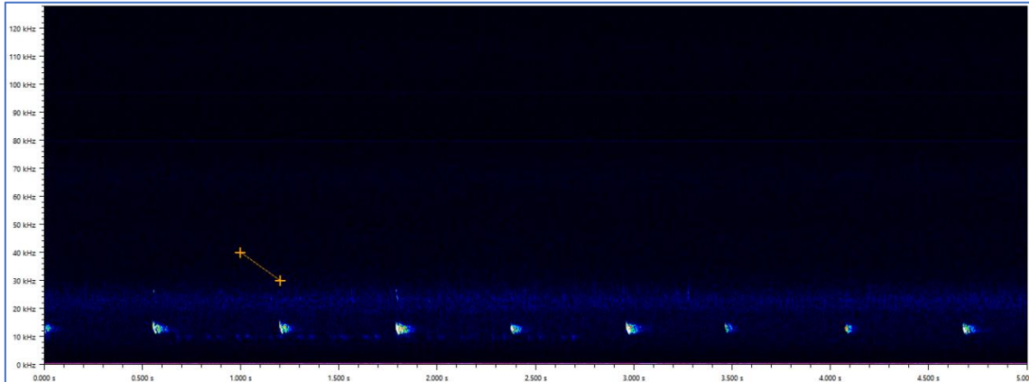
Figura 37. Sonograma de murciélago rabudo ( Tadarida teniotis ) Fuente propia
