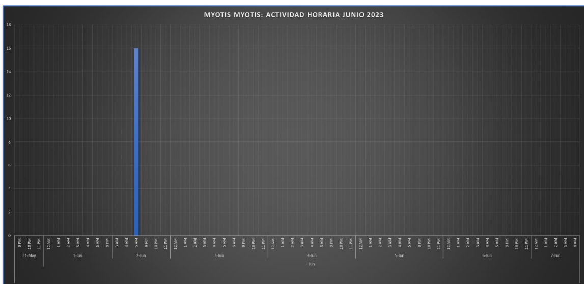
Figura 18. Actividad horaria junio del grupo fónico Myotis myotis . Fuente propia
