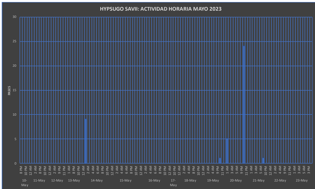
Figura 23. Actividad horaria en mayo de Hypsugo savii . Fuente propia
