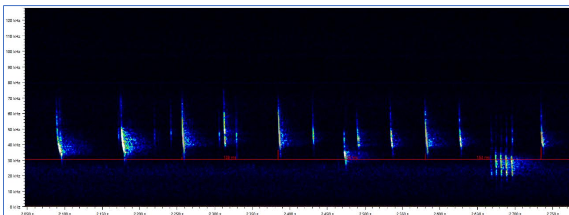
Figura 14. Sonograma perteneciente al grupo fónico Myotis 30 que incluye, además, llamada social. Fuente propia
