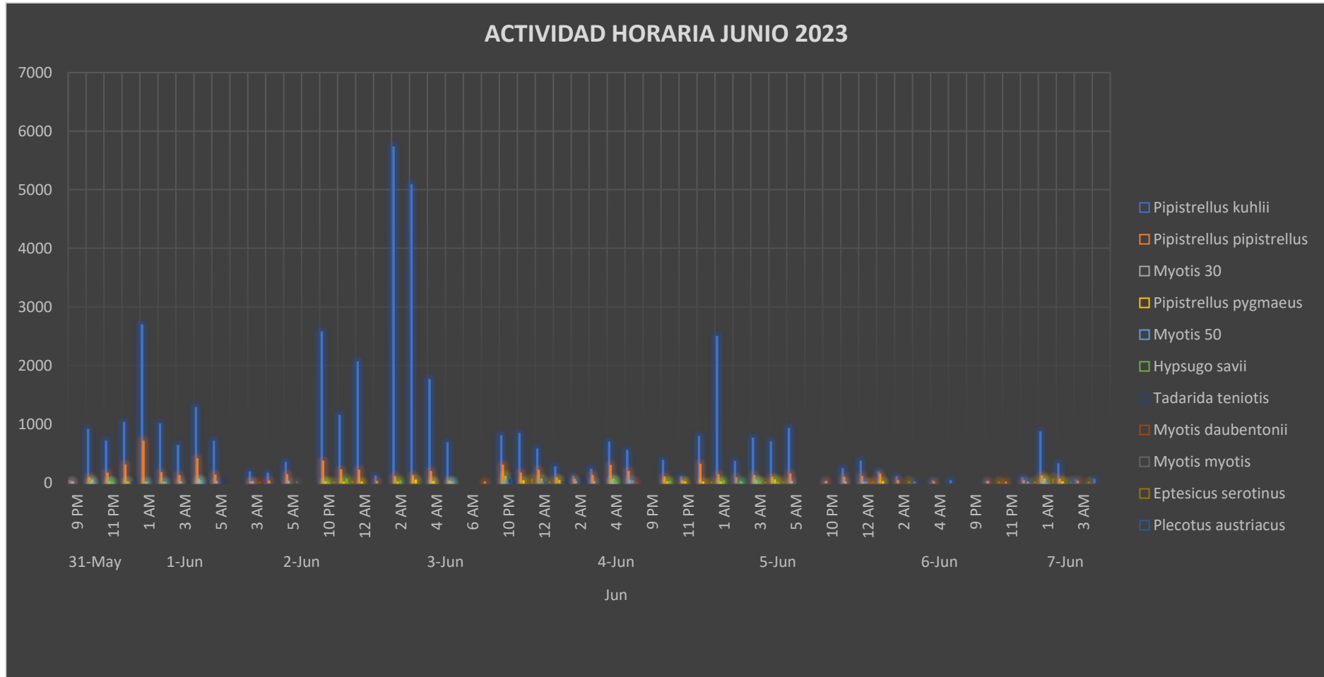
Figura 45. Distribución horaria de los registros obtenidos en la sesión del mes de junio de 2023 en la estación de ultrasonidos. Fuente propia
