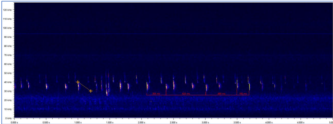
Figura 20. Sonograma perteneciente al grupo fónico Murciélago ratonero ribereño ( Myotis daubentonii ). Fuente propia
