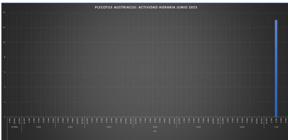
Figura 36. Actividad horaria de junio de Plecotus austriacus . Fuente propia
