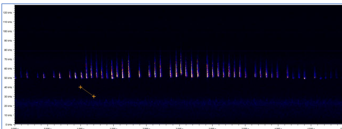
Figura 31. Sonograma de murciélago de Cabrera ( Pipistrellus pygmaeus ) Fuente propia
